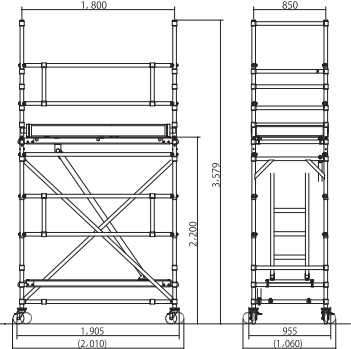
作業床高さ2200mm状態
