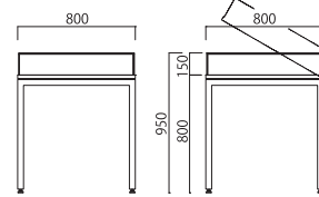
展示ケース・STF-8080
