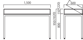
展示ケース・STF-15060 (15060-2)
