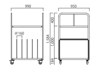
折たたみ式展示台座用台車 NT-TUD-6
