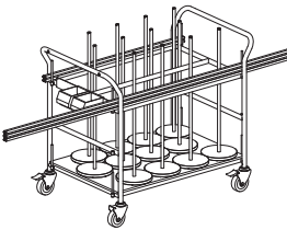
NT-WGK-3 (フレキシブル75・フラットバー72タイプ)
